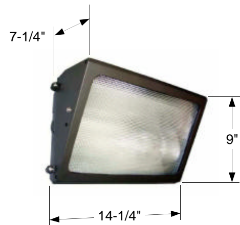
QPE15 Max. 175W MH or 150W HPS or 2-PLT42W CF
